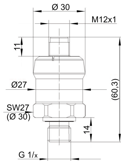
Ausführung DLF...A
