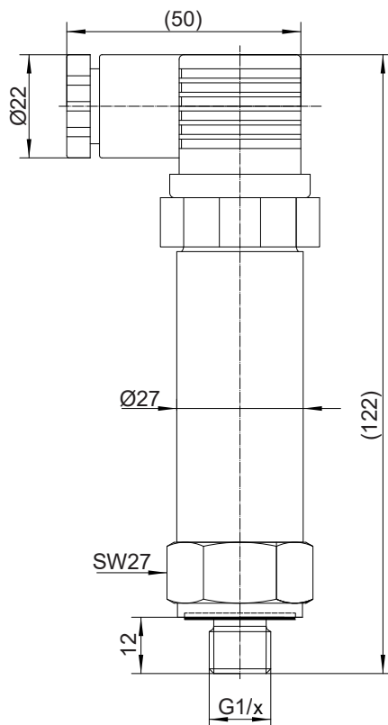
Ausführung DLF...V
