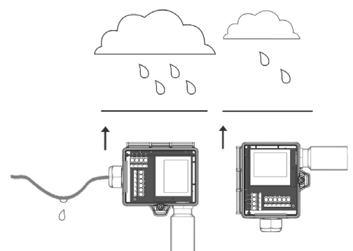
Kabelzuführung
